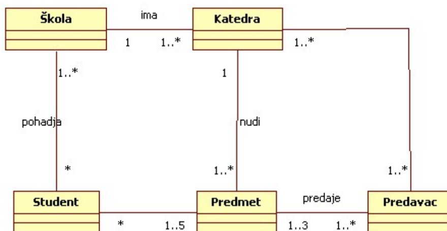
Slika 1 - Izgled traženog dijagrama klase
