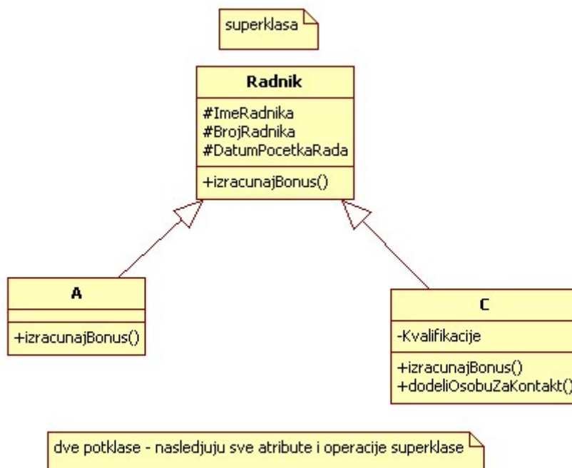
Slika 1 - Izgled traženog dijagrama klase
