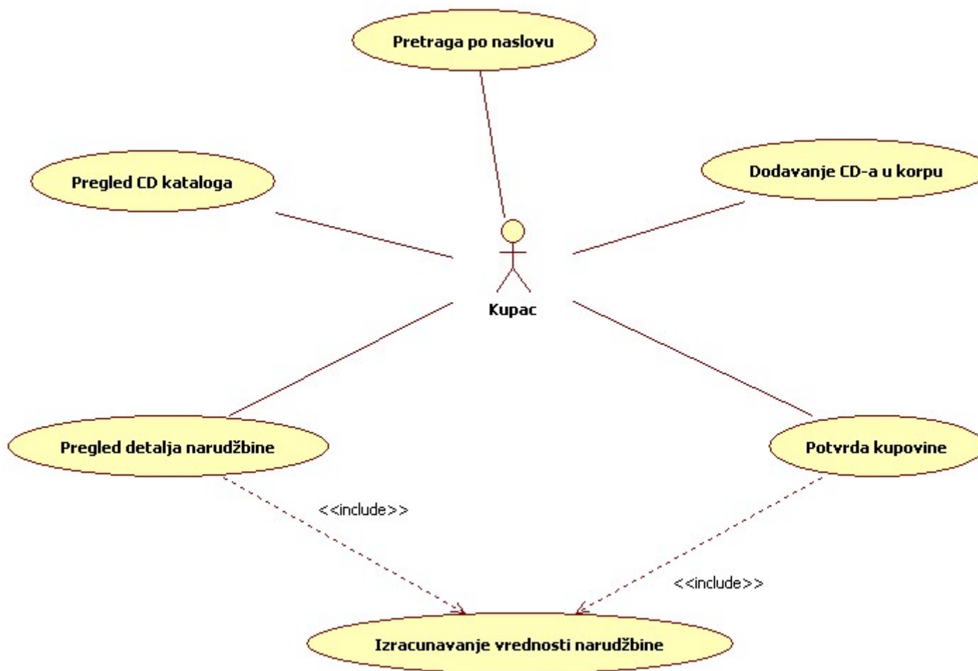
Slika 2 - Izgled traženog dijagrama slučaja korišćenja
