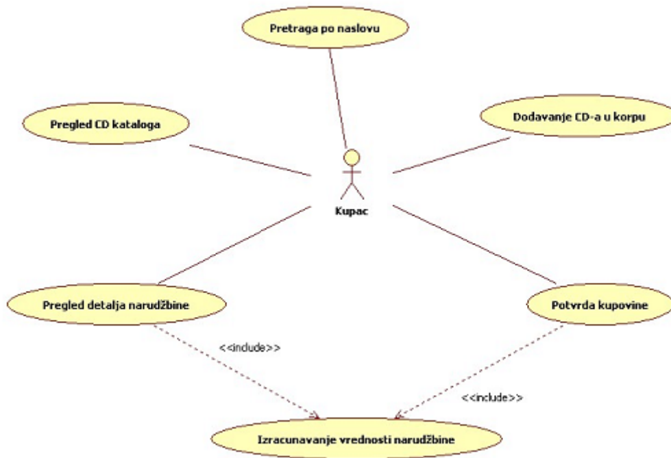
Slika 1 - Izgled traženog dijagrama slučaja korišćenja (kliknite za uvećan prikaz)
